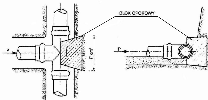
BŁOK OPOROWY TRÓJNIKA
