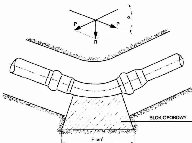
BŁOK OPOROWY KOLANA LUB ŁUKU
