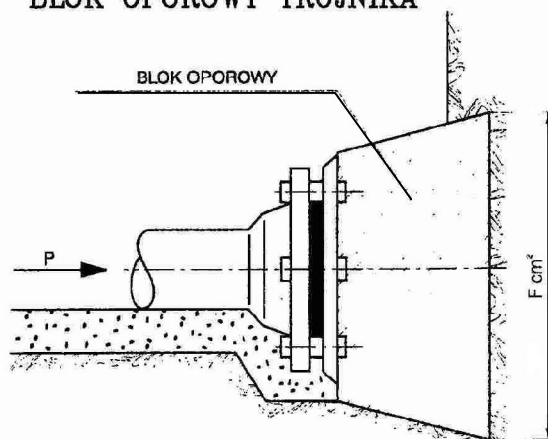
BŁOK OPOROWY KORKA NA KONCÓWCE PRZEWODU
